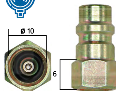
Tipo: Válvula de Carga 1/4
