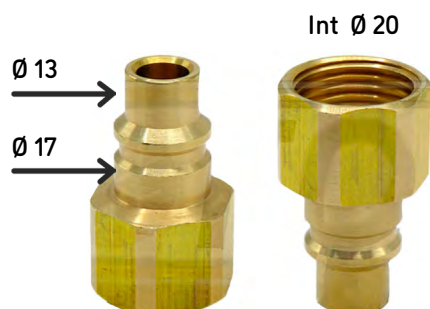
Tipo: Adaptador Botija Referências Originais: APFR200033, APFR200029
